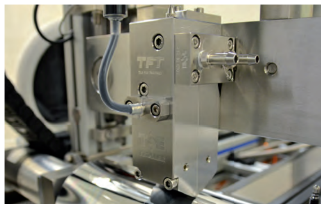
Schlitzdüsenbeschichtung an der Hochpräzisions-schlitzzußanlage
