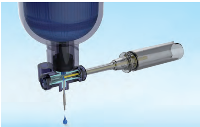
Illustration eines im Projekt entwickelten Dispensers.
